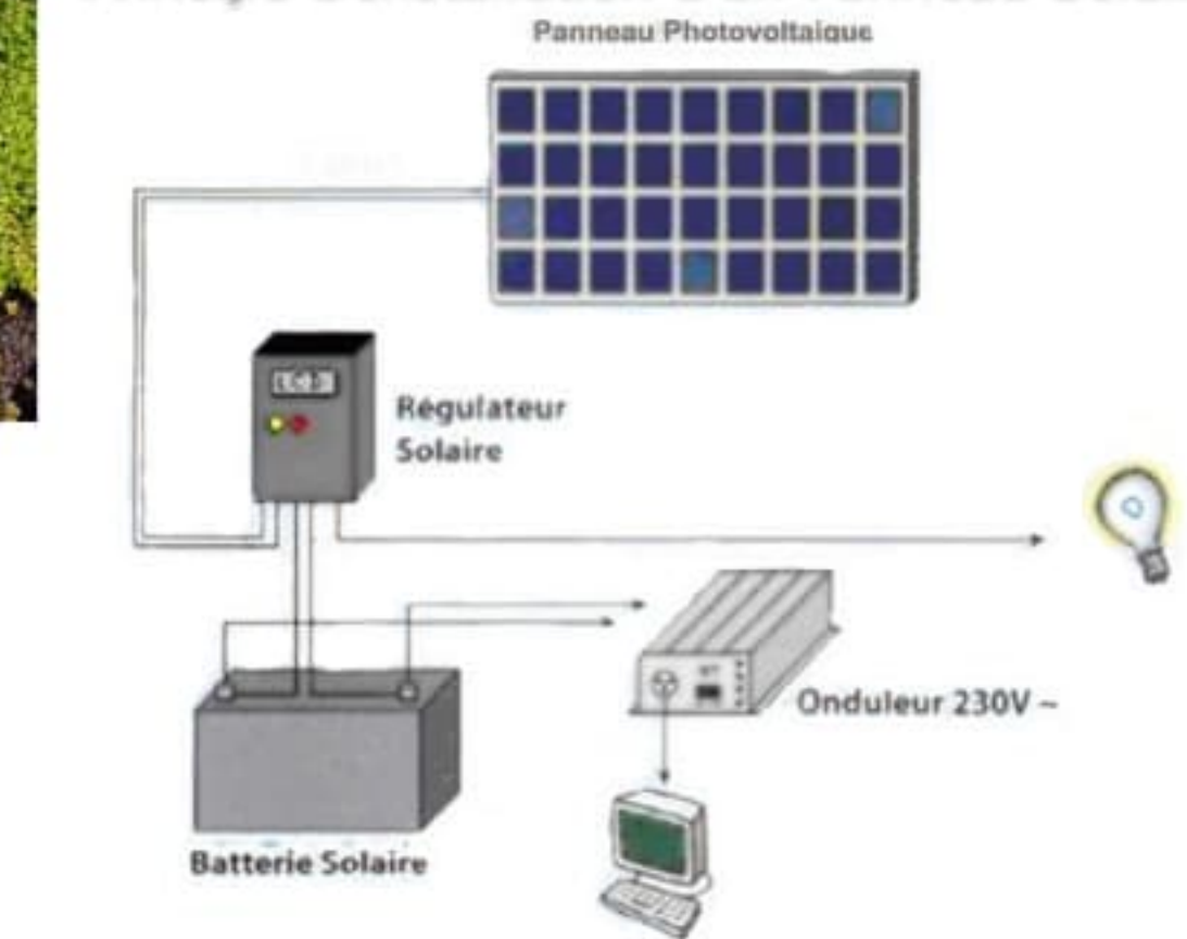
Principe d'Installation d'un Panneau Solaire
